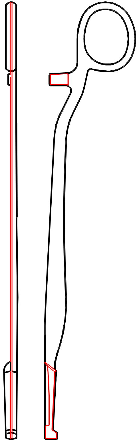
0118-000 Mikuliczklemme 20 cm aufgelegt Ring klein
