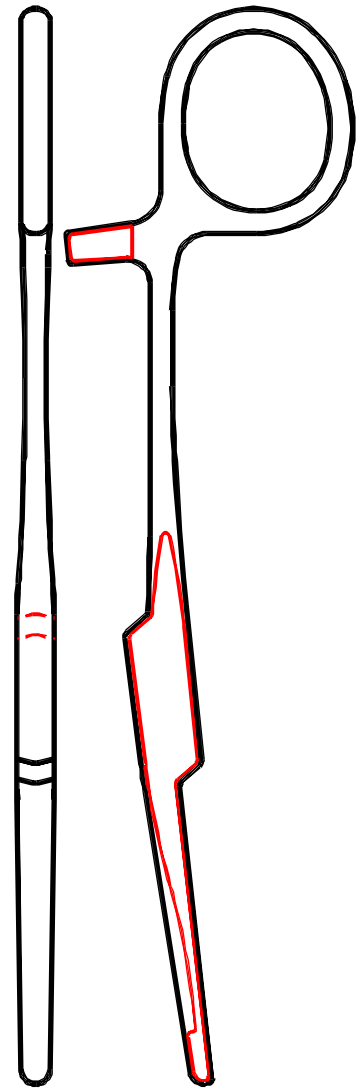
0267-000 Pean 14 cm langfassend
