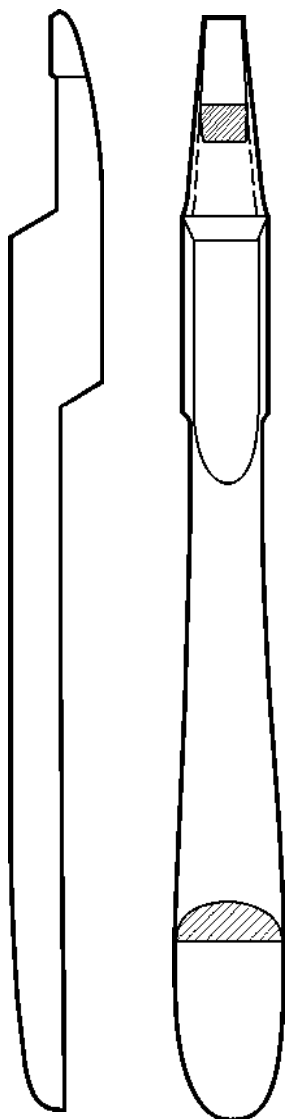
0618-000 Biegezange 14 cm
