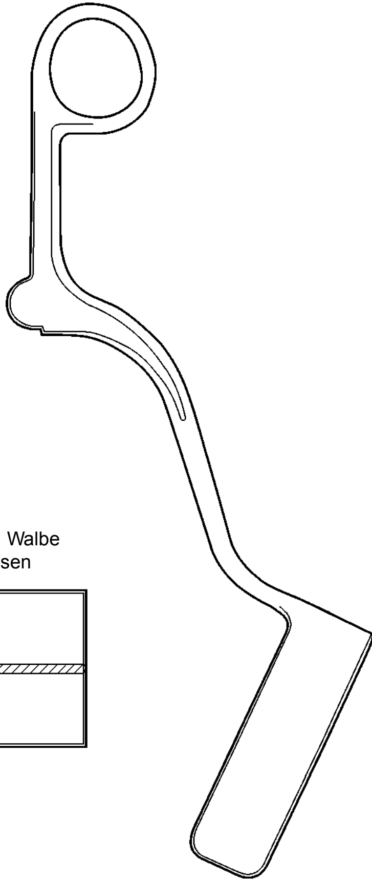
3010-000 Wundsperrer Rigby 19 cm
